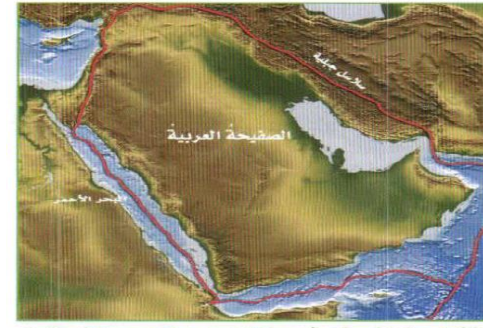
تكوّن البحر الأحمر عن حركة الصفيحة العربية في اتجاه الشمال الشرقي.
